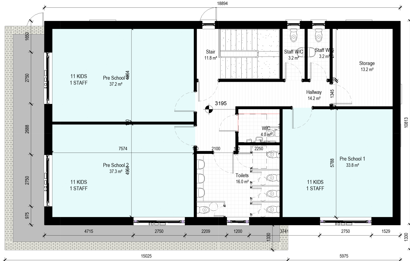
2: BX01 Creche - L01 First Floor Plan Scale - 1 : 100
